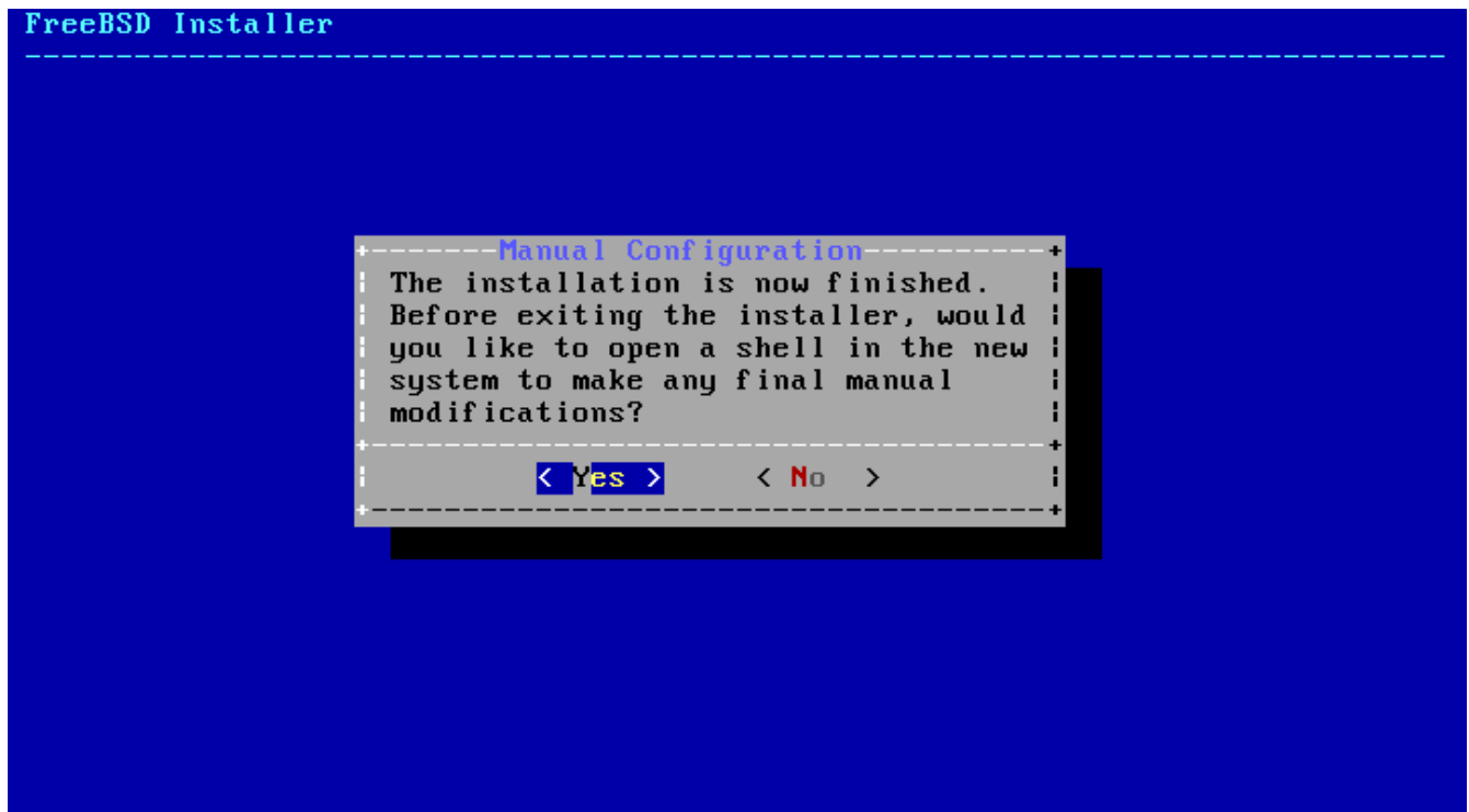
図 58. Manual Configuration
