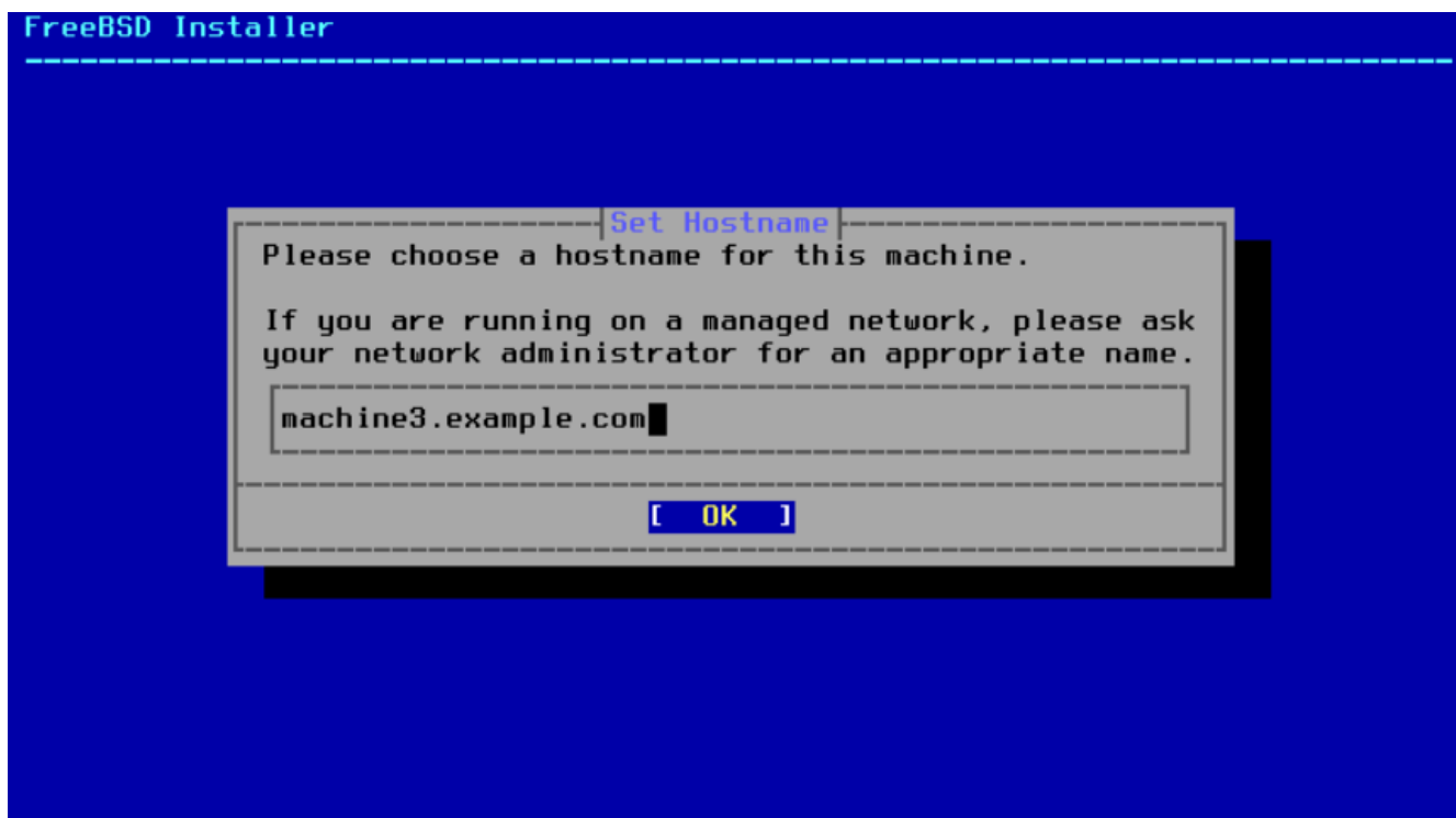
Figura 7. Configurando o nome do host
