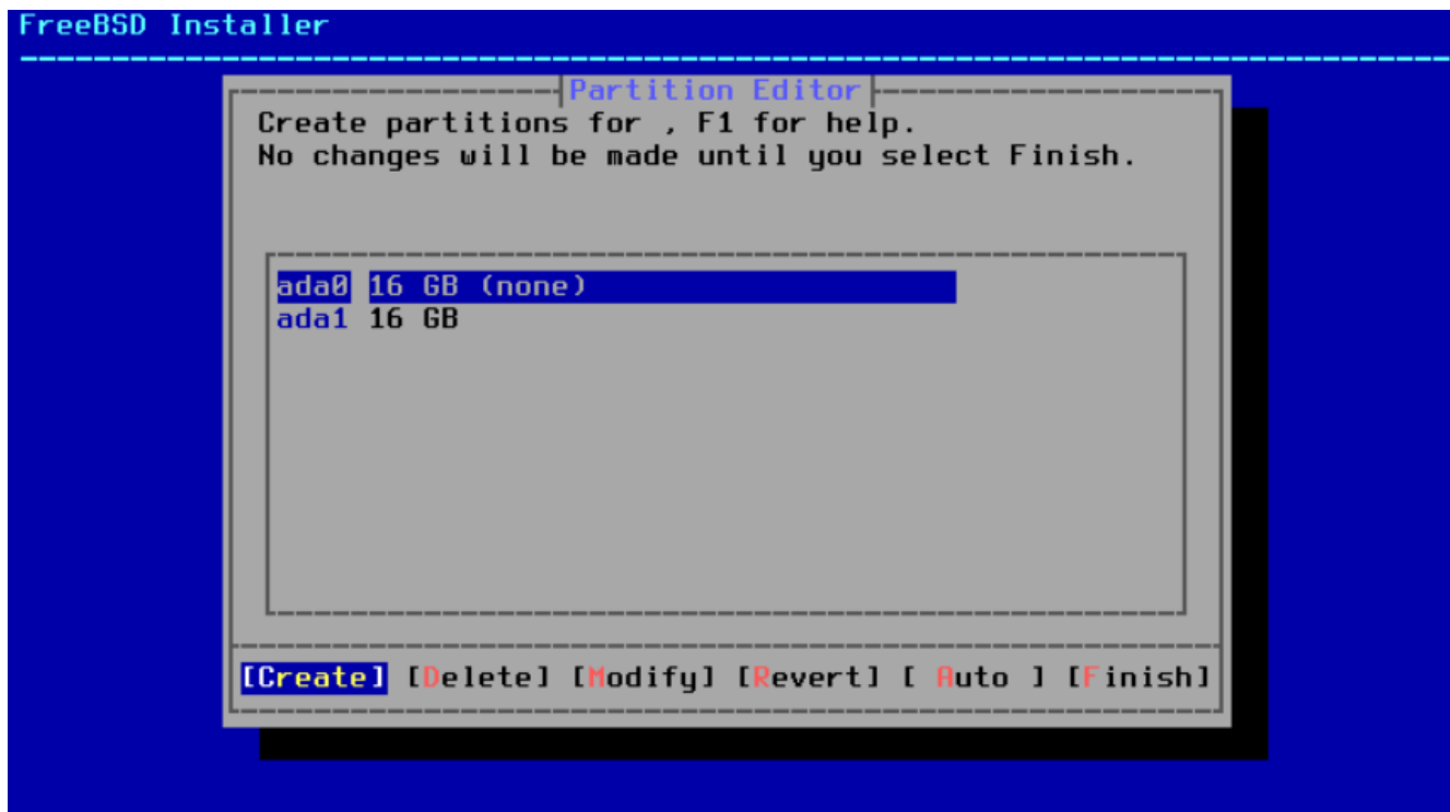
Figura 17. Criar partições manualmente
