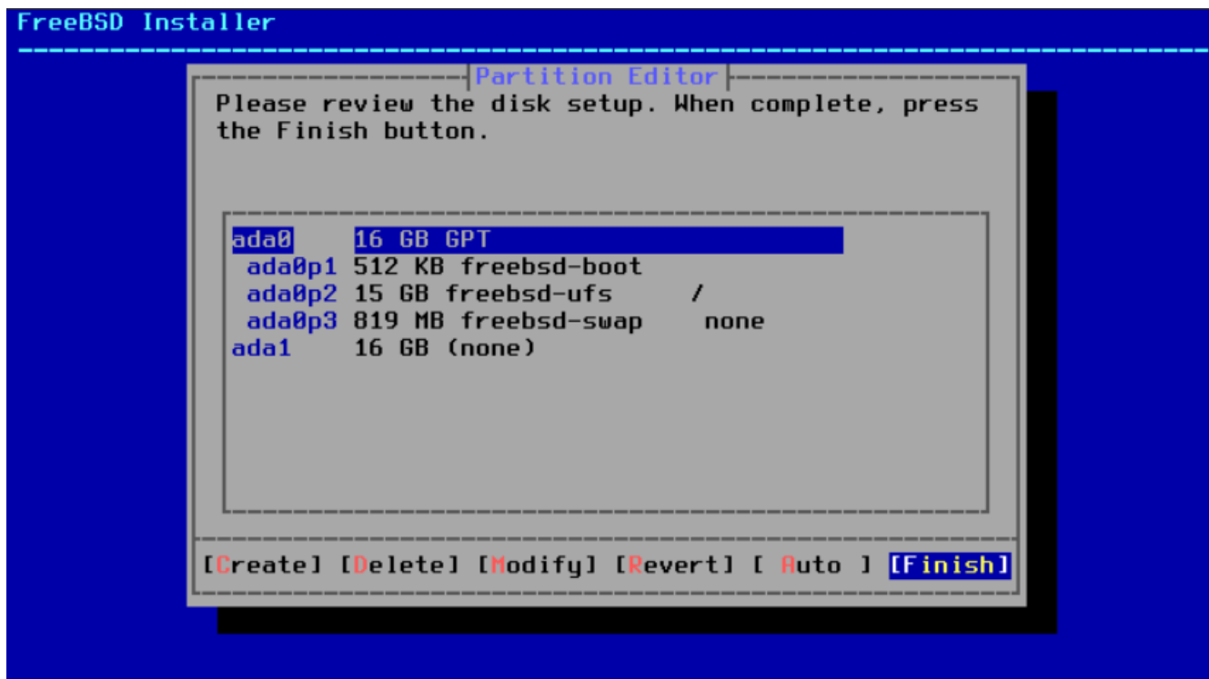
Figura 15. Revise as partições criadas
